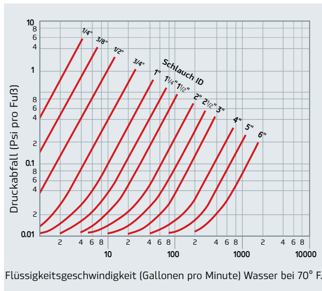
Druckabfall-Diagramm für Wasser
