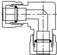
765 UH WINKELVERSCHRAUBUNG
