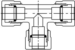
764 UH T-VERSCHRAUBUNG
